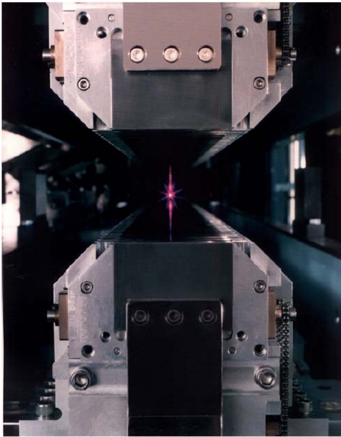
ALS U5 undulator, beamline 7.0, N = 89 , \lambda_u = 50 mm
